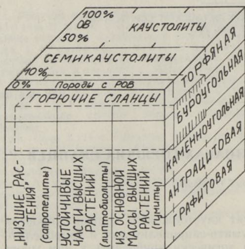
Рис. 2. Породы с РОВ, горючие сланцы и угли, разграниченные по содержанию в них ОВ, первичной биопродукции и степени преобразования ОВ. Боковая грань блока «горючие сланцы» оттенена.
