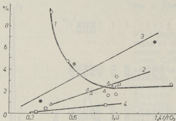
Рис. 2. Выход газообразного водорода в % от исходного водорода органического вещества каустобиолита в зависимости от расхода кислорода ( g/g ). 1 — каменный уголь Фан-Ягнобского месторождения, 2 — бурый уголь Ангренского месторождения, 3 — кукерсит при 270 °С, 4 — кукерсит при 175 °С.
