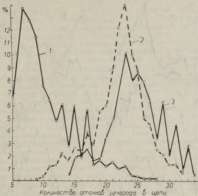
Рис. 1. Состав n -парафинов и n -парафиновых цепей органического вещества составляющих геосферы Северной Эстонии. 1 — n -парафиновые цепи керогена кукуерсита, установленные способом термической деструкции, 2 — n -парафины битумоида кукуерсита, 3 — n -парафины шахтных вод.
