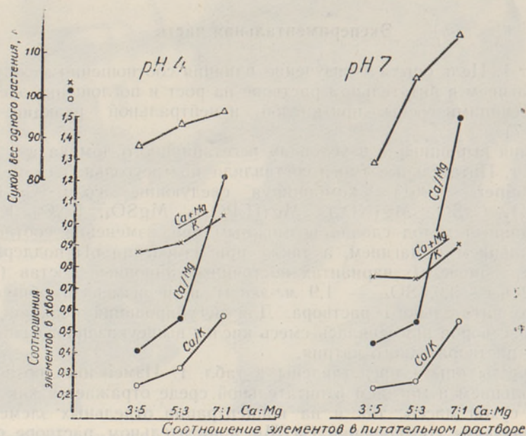
Рис. 3. Влияние соотношения Ca/Mg в питательном растворе на рост сеянцев и соотношение элементов в хвое (высчитаны по содержанию элементов в мг-экв/100 г). Опыт 1.
