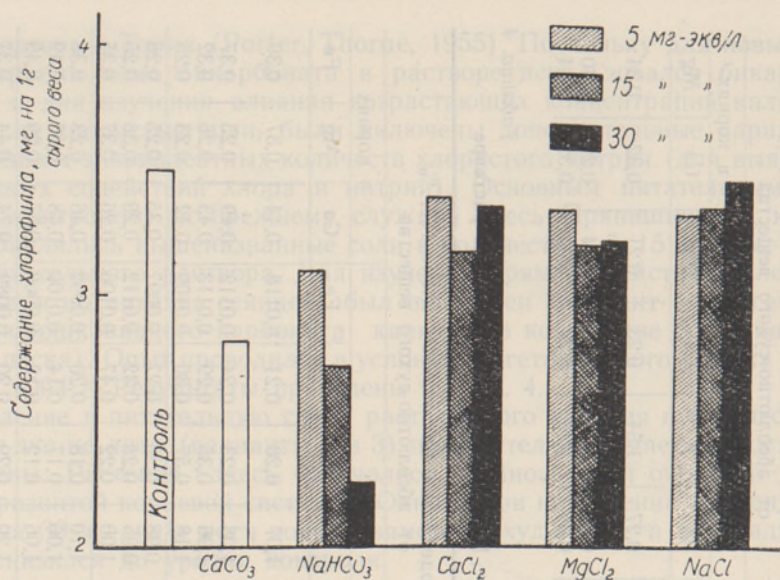
Рис. 6. Влияние \text{CaCO}_3 , \text{NaHCO}_3 , \text{CaCl}_2 , \text{MgCl}_2 и \text{NaCl} на содержание хлорофилла в хвое. Опыт 4.
