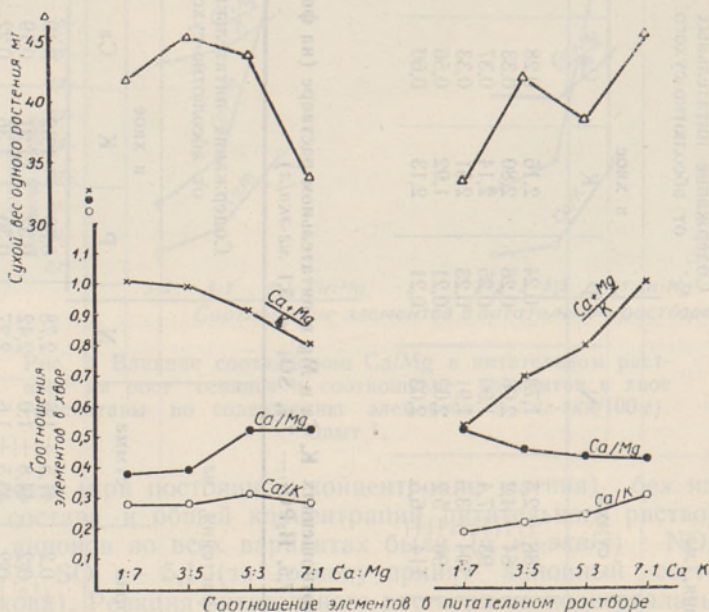
Рис. 4. Влияние соотношений Ca/Mg и Ca/K в питательном растворе на рост сеянцев и соотношение элементов в хвое (высчитаны по содержанию элементов в мг-экв/100 г). Опыт 2.
