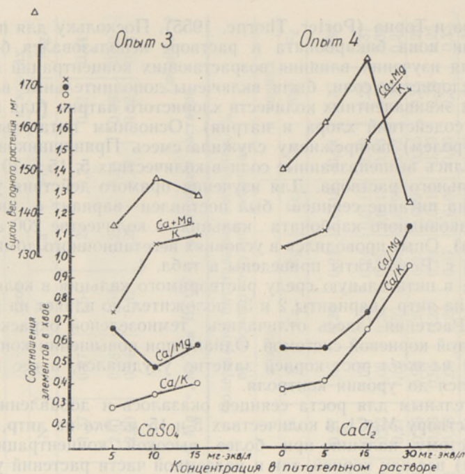
Рис. 5. Влияние концентраций \text{CaSO}_4 (опыт 3) и \text{CaCl}_2 (опыт 4) в питательном растворе на рост сеянцев и соотношение элементов в хвое (высчитаны по содержанию элементов в мг-экв/100 г).
