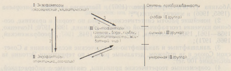
Рис. 1. Группировка природных факторов по структурно-генетическому принципу и теоретико-методическая очередность в ландшафтных исследованиях.
