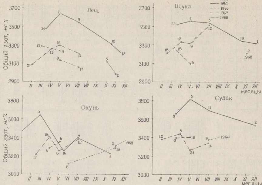
Сезонная динамика содержания общего азота в мышцах изученных видов рыб; ..... 1964 г., — 1965 г., - - - 1966 г., — · — · 1968 г.
