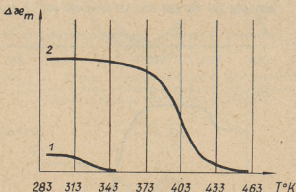
Рис. 9. Кривые термообесцвечивания рентгенизированного KCl : 1 — в M -полосе добавочного поглощения (825 мкм), 2 — в F -полосе добавочного поглощения (555 мкм).
