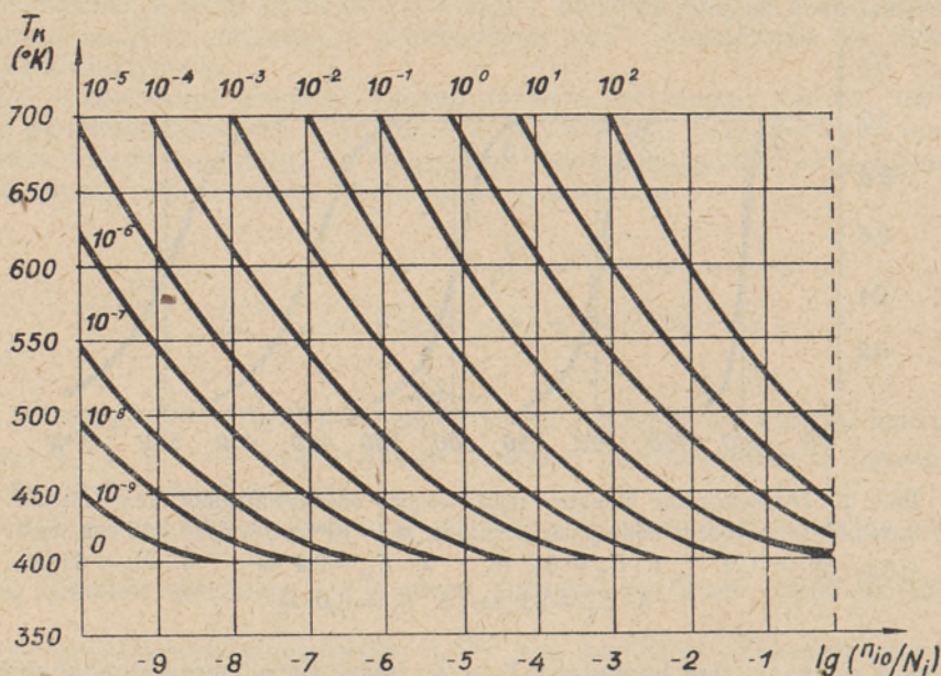
Рис. 3. Теоретическая зависимость T_k от числа запасенных электронов при различных \gamma = \sigma_s/\sigma_p ( E_T = 1,0 эв, \rho_0 = 10^{10} сек ^{-1} , \beta_0 = 0,15 град/сек, \delta_k = 20^\circ К).
