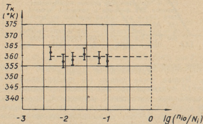
Рис. 10. Зависимость T_k кривых термообесцвечивания для Z_1 -полосы поглощения (580 мкм) в KCl \cdot CaCl_2 от числа запасенных электронов.
