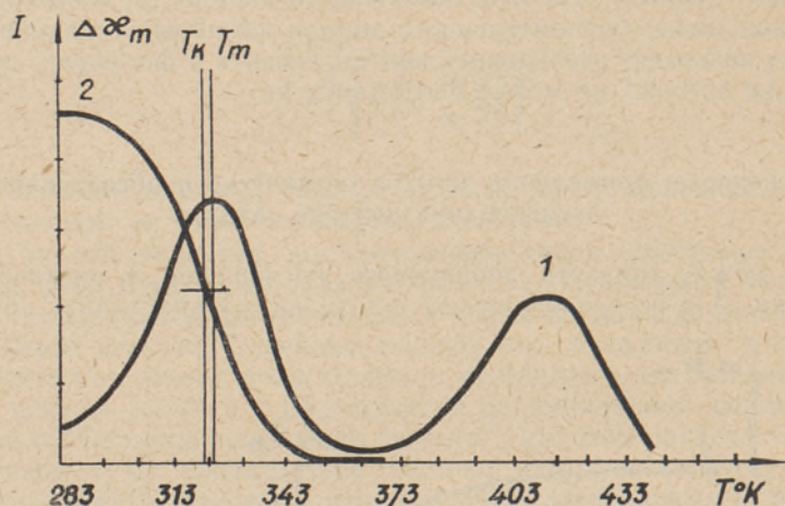
Рис. 5. 1 — Кривая термовысвечивания рентгенизированного \text{KCl} \cdot \text{TlCl} , 2 — кривая термообесвечивания рентгенизированного \text{KCl} для M -полосы поглощения (825 мкм).
