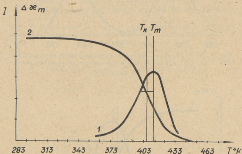
Рис. 4. 1 — Кривая термовысвечивания KCl \cdot TlCl (предварительно прогрет до 380^{\circ}K ), 2 — кривая термообесцвечивания рентгенизированного KCl для F -полосы поглощения (555 мкм).
