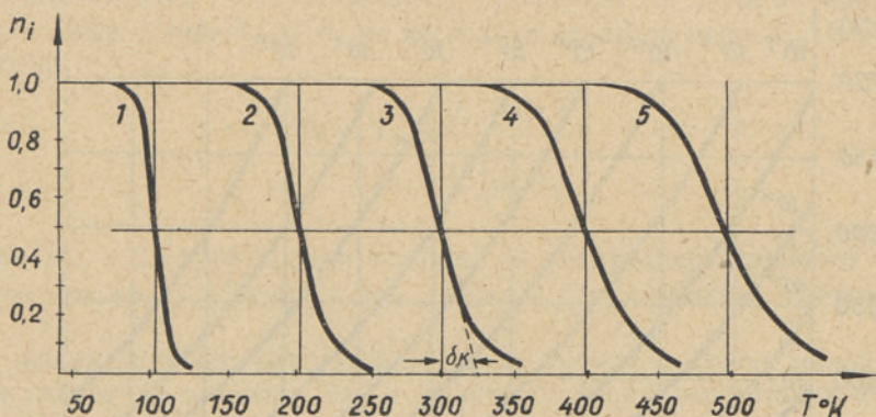
Рис. 1. Теоретические кривые термического обесцвечивания для случая большой вероятности повторных захватов. \rho_0 = 10^{10} сек ^{-1} , \beta_0 = 0,15 град/сек, \sigma_p n_{i0} / \sigma_3 N_i = 0,01 . 1. E_T = 0,2 эв, 2. E_T = 0,4 эв, 3. E_T = 0,6 эв, 4. E_T = 0,8 эв, 5. E_T = 1,0 эв.
