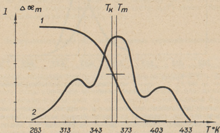
Рис. 6. 1 — Кривая термообесвечивания \text{KCl} \cdot \text{CaCl}_2 для Z_1 -полосы поглощения (580 мкм), 2 — кривая термовысвечивания рентгенизированного \text{KCl} \cdot \text{CaCl}_2 \cdot \text{TlCl} .
