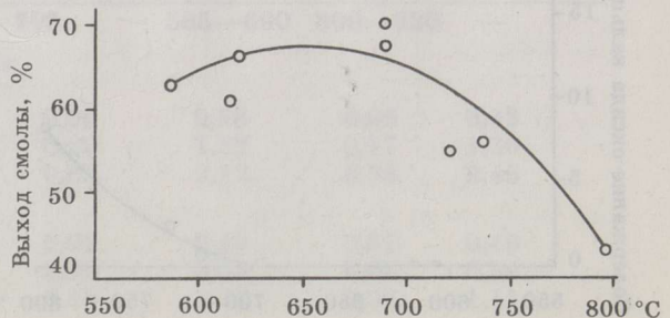
Рис. 1 Зависимость выхода смолы (%) от температуры в технологической топке
